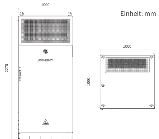
Toleranz: Länge ±2mm, Breite ±2mm
