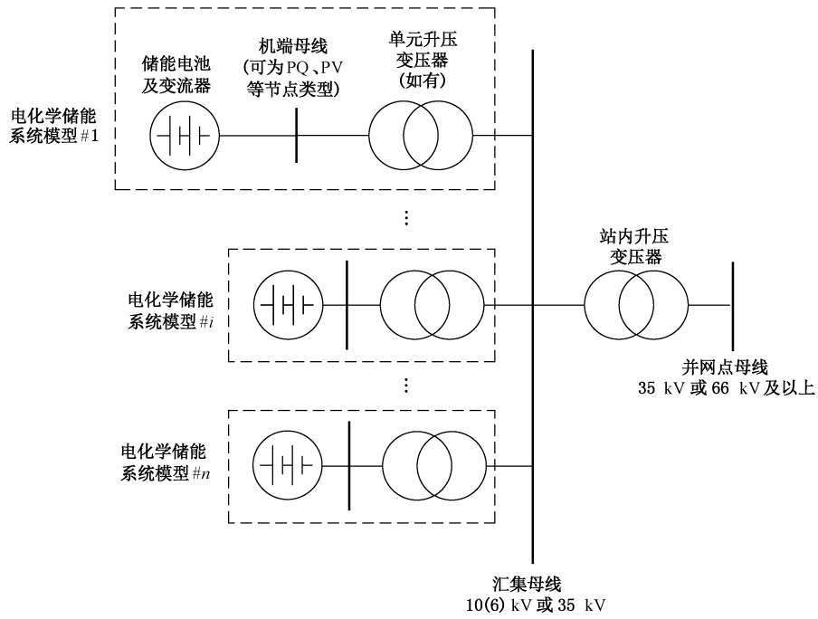
图 B.1 电化学储能电站潮流计算模型结构图
