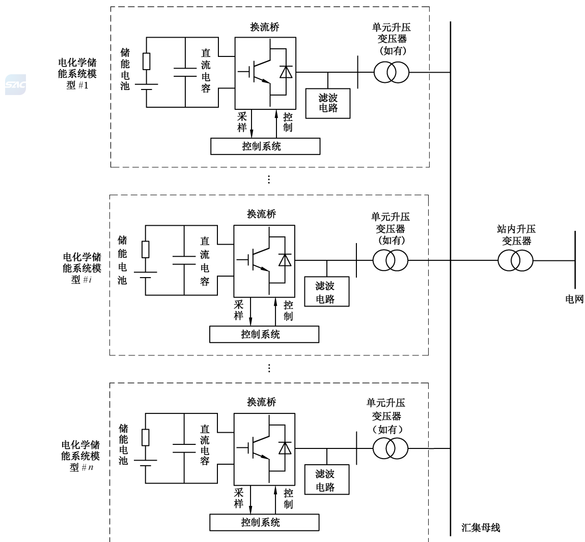
图 C.1 电化学储能电站电磁暂态仿真模型典型结构图
