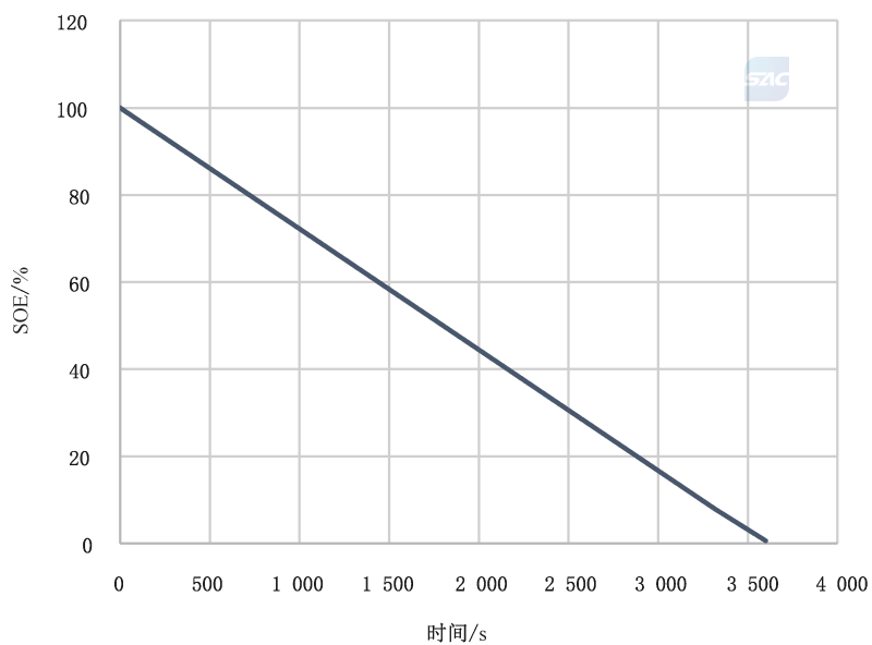
图 D.4 电池放电 SOE-时间曲线
