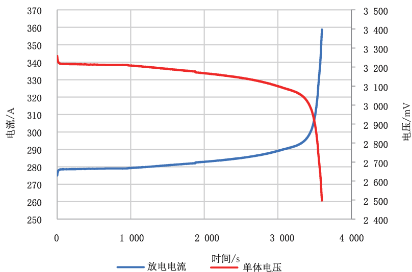
图 D.3 电池放电 V_{dis}/I_{dis} -时间曲线
