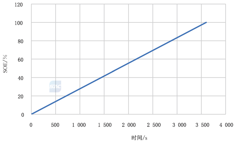
图 D.2 电池充电 SOE-时间曲线
