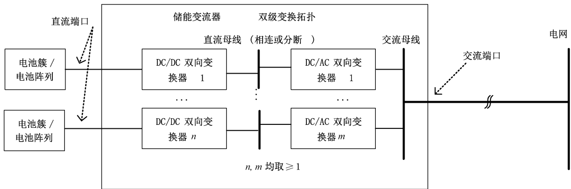
图 A.2 双级变换架构典型拓扑
