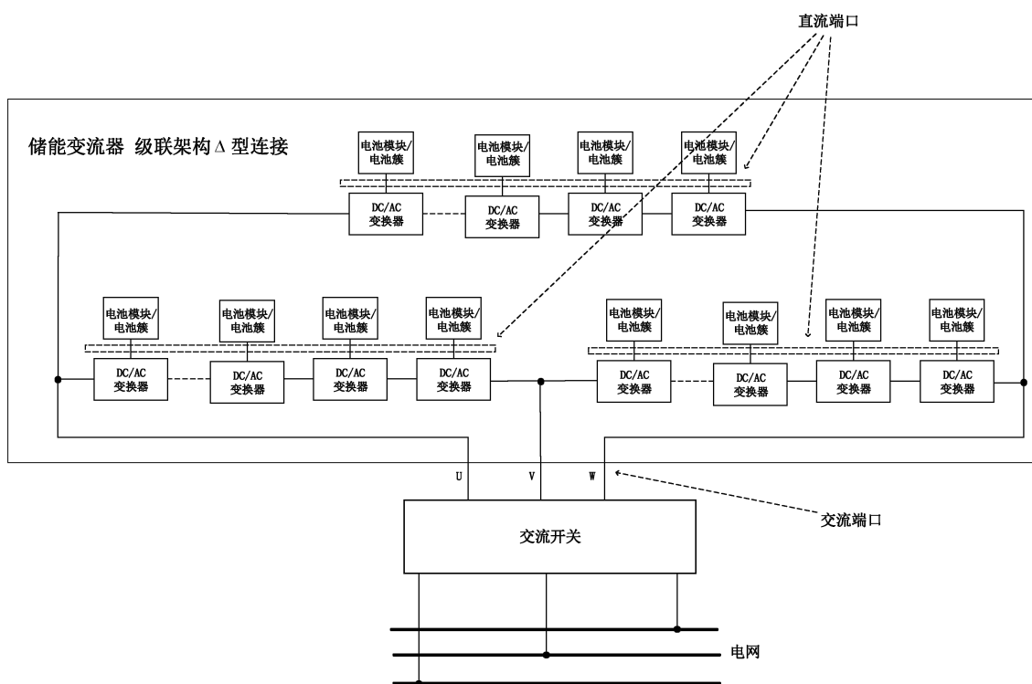
图 A.4 级联架构典型拓扑- \Delta 型连接
