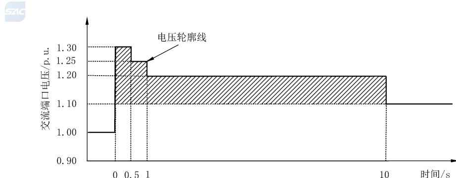
图 5 储能变流器高电压穿越能力要求
