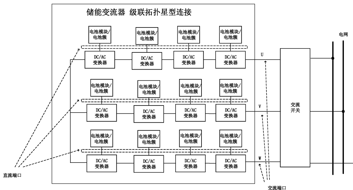
图 A.3 级联架构典型拓扑-星型连接
